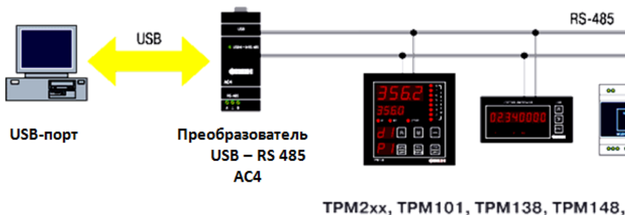
Рис.1. Схема подключения контрольно-измерительных и управляющих приборов для работы с SCADA системой
