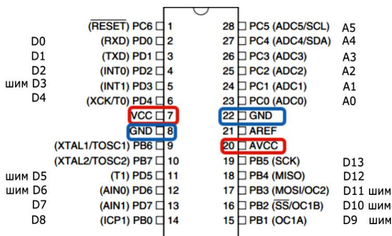
Рис.4. Расположение входов и выходов GPIO МК Atmega328
