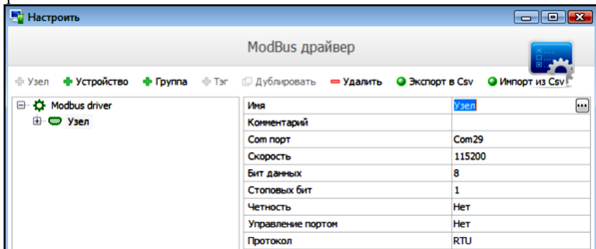
Рис.5. Настройка узла
