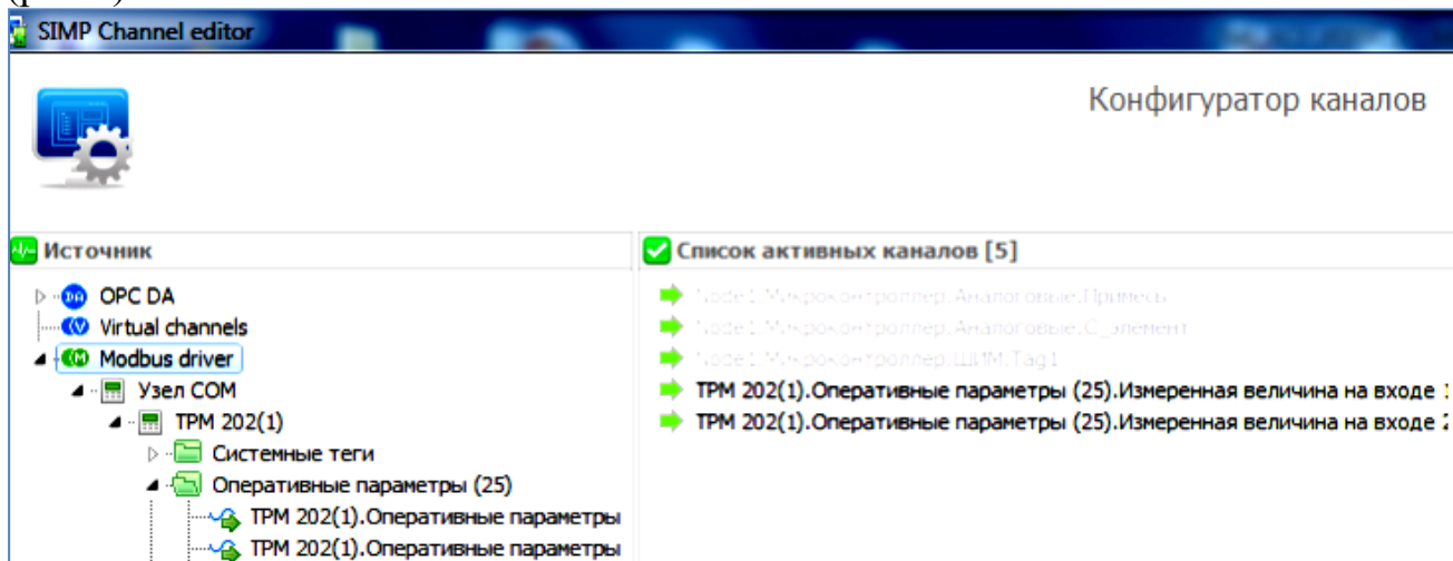
Рис.8. Пример создания списка активных каналов.
