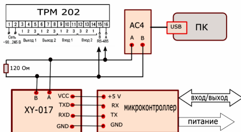
Рис.2. Схема подключения приборов к компьютеру по линии RS485.
