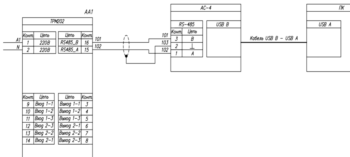
Рис.5. Схема подключения измерителя-регулятора TPM202 и преобразователя интерфейса А4 к компьютеру.
