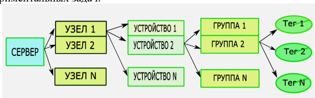
Рис. 2. Структура дерева объектов интерфейса OPC сервера
