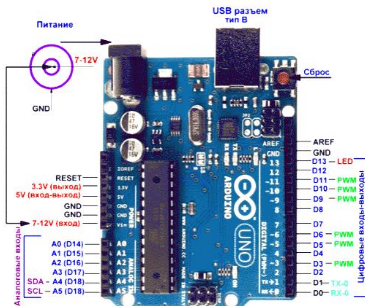
Рис.5. Плата Arduino Uno
