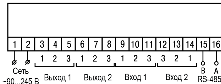
Рис.3. Схема контактов тыловой части измерителя-регулятора ОВЕН ТРМ202
