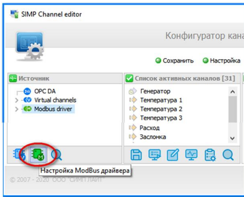
Рис.2. Вызов Modbus drive
