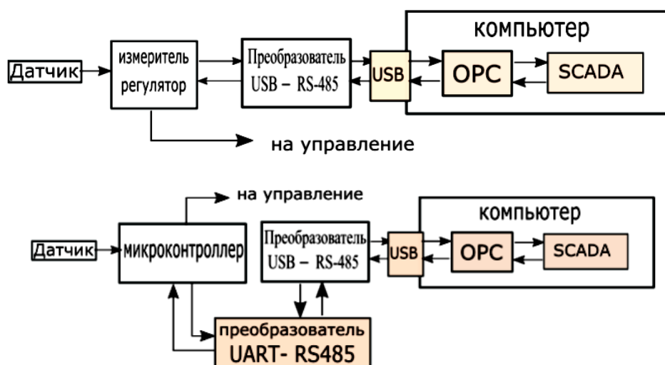
Рис. 1. Схемы сопряжения физического уровня с программным обеспечением
