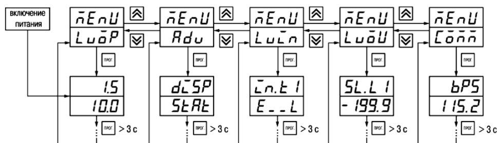
Рис. 7. Навигация в меню настройки ОВЕН ТРМ 202
