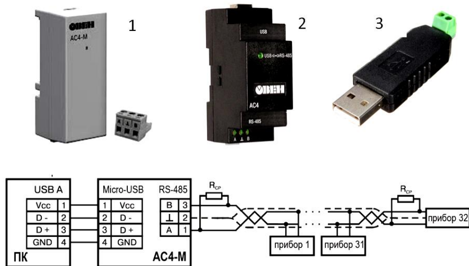
Рис.4. Преобразователи интерфейса USB – RS485 и способ их соединения.
