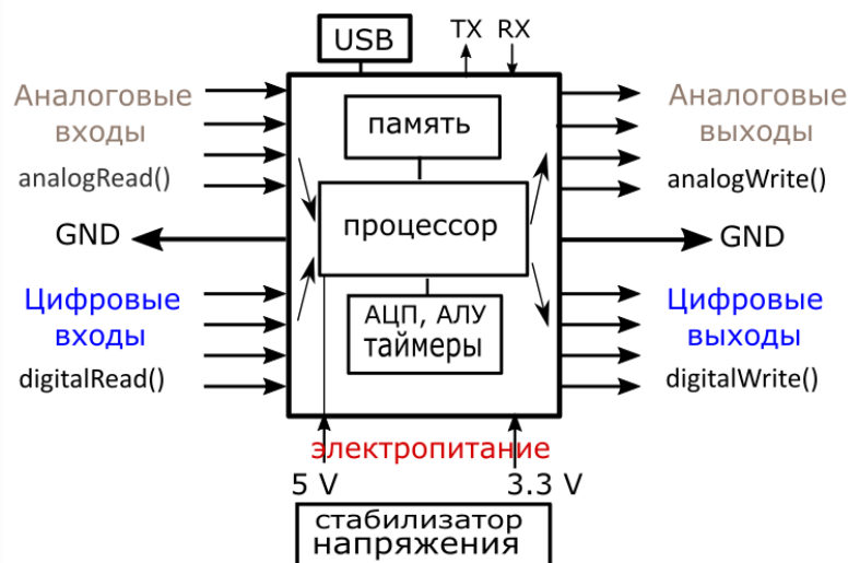
Рис.3. Схематический интерфейс платы содержащей микроконтроллер
